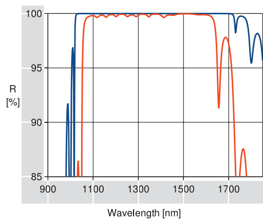
BROADBAND H.R. COATING R67: 1100-1600nm S-POL, 45° ———— P-POL, 45° ————
