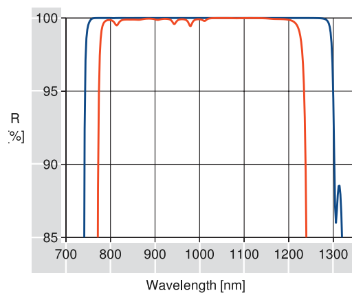
BROADBAND H.R. COATING R66: 800-1200nm S-POL, 45° ———— P-POL, 45° ————
