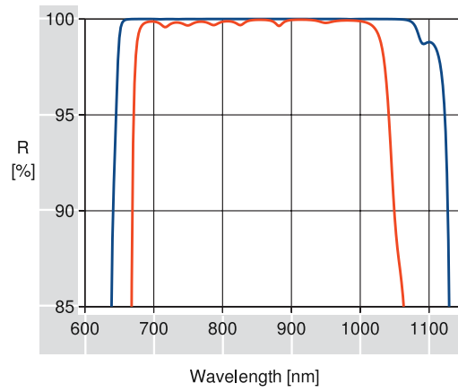
BROADBAND H.R. COATING R62: 700-1000nm S-POL, 45° ———— P-POL, 45° ————
