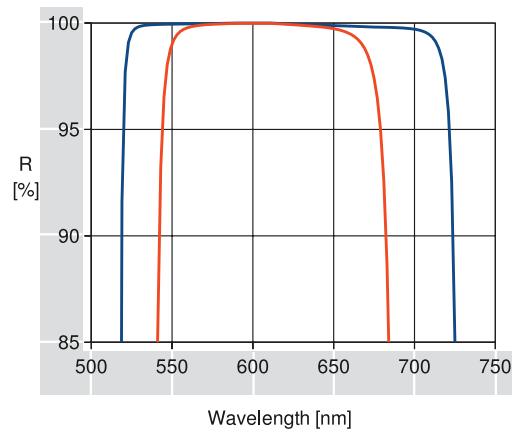
BROADBAND H.R. COATING R61: 570-640nm S-POL, 45° ———— P-POL, 45° ————
