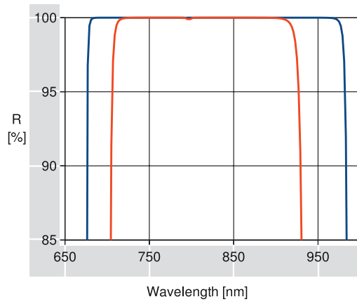
BROADBAND H.R. COATING R60: 730-900nm S-POL, 45° ———— P-POL, 45° ————
