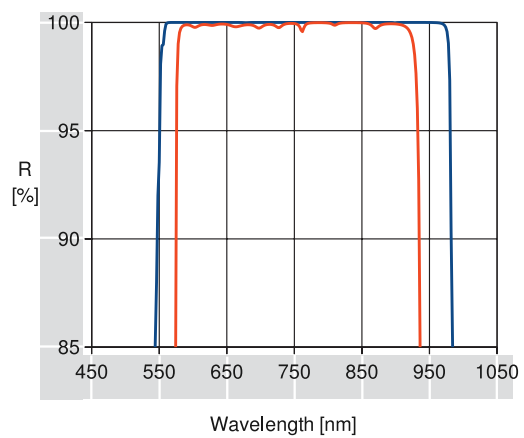
BROADBAND H.R. COATING R58: 600-900nm S-POL, 45° ———— P-POL, 45° ————
