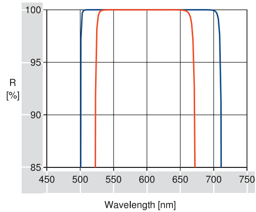
BROADBAND H.R. COATING R57: 540-650nm S-POL, 45° ———— P-POL, 45° ————
