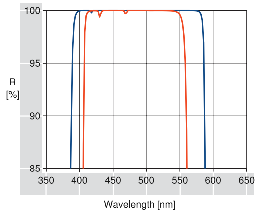
BROADBAND H.R. COATING R56: 420-540nm S-POL, 45° ———— P-POL, 45° ————
