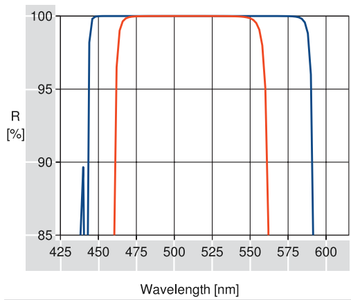
BROADBAND H.R. COATING R53: 480-540nm S-POL, 45° ———— P-POL, 45° ————
