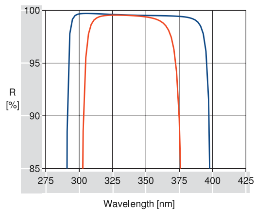
NARROWBAND H.R. COATING R09: 335nm S-POL, 45° ———— P-POL, 45° ————
